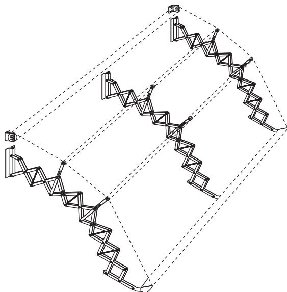
■アルミ前枠式(連装) (サポートパイプ4本又は6本付)
