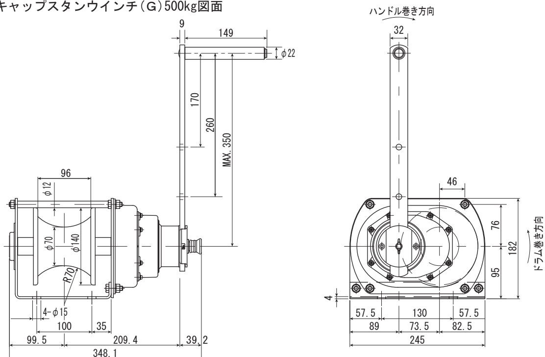
■キャップスタンウインチ(G)500kg図面
