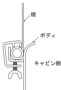
側面納まり図
