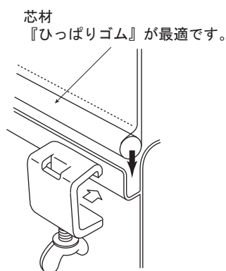
取付図
