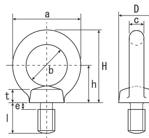
●IB-6・8・10・12・16の寸法図
