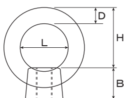
●IN-4・5の寸法図
