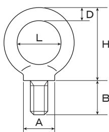
●IB-4・5の寸法図
