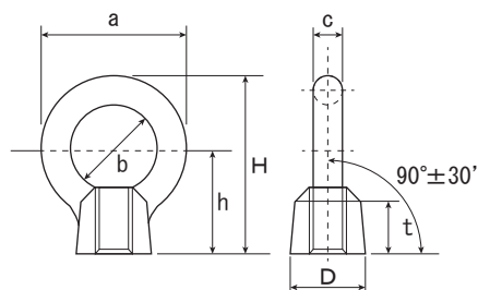
●IN-6・8・10・12・16の寸法図
