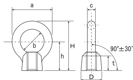
●IN-6・8・10・12・16の寸法図
