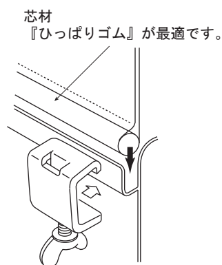
取付図
